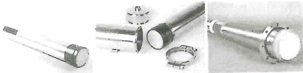
SEPURAN® Green Cartouche : Cartouche (Housse & bride) cartouche dans la housse
